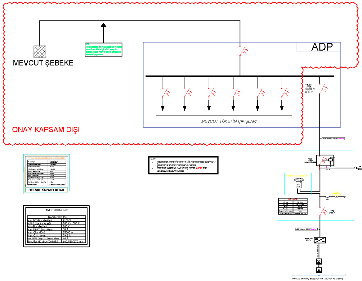
Şekil 3. Tek Hat Şeması
